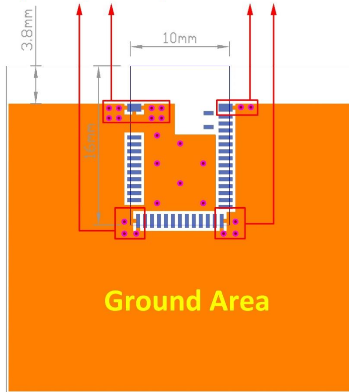
Top layer
