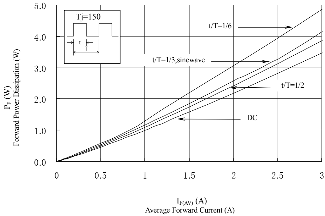
I_{F(AV)} - P_F
