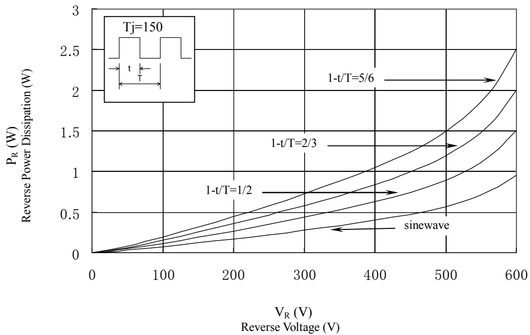
V_R - P_R
