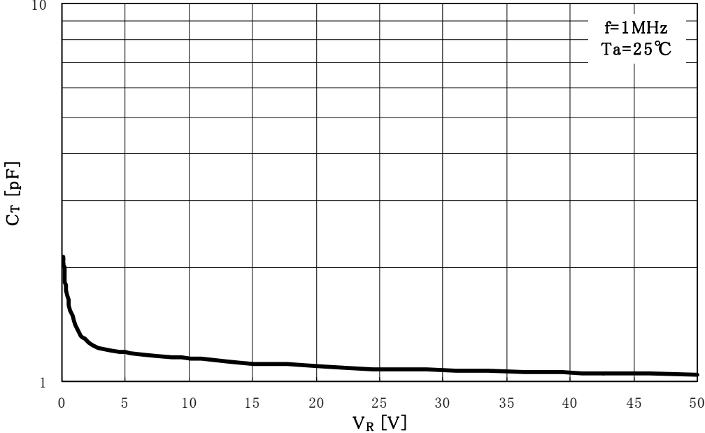
C_T-V_R
